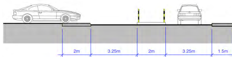
Fig. 3 - Variante A: apertura dello spartitraffico di fronte all'uscita del posteggio Coop
