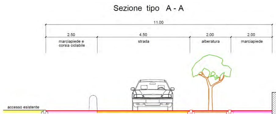
Fig. 1 - Sezione tipo A-A del tratto di strada rinnovato
