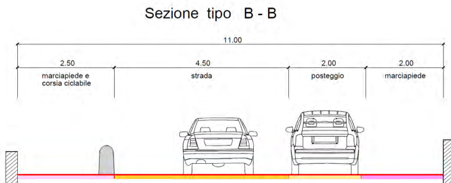
Fig. 2 - Sezione tipo B-B del tratto di strada rinnovato
