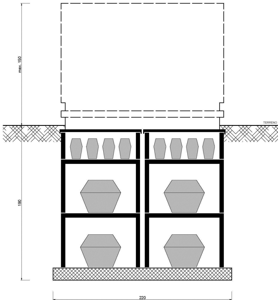
SEPOLCRO DI FAMIGLIA DOPPIO (TIPO B) VISTA FRONTALE
