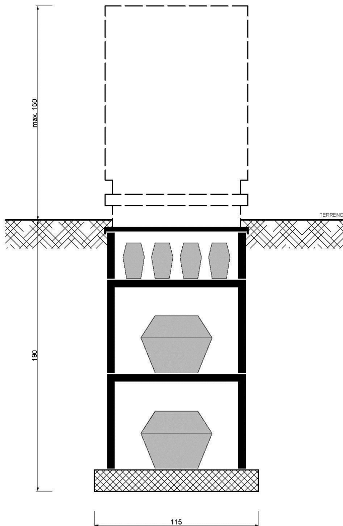
SEPOLCRO DI FAMIGLIA SEMPLICE (TIPO A) VISTA FRONTALE
