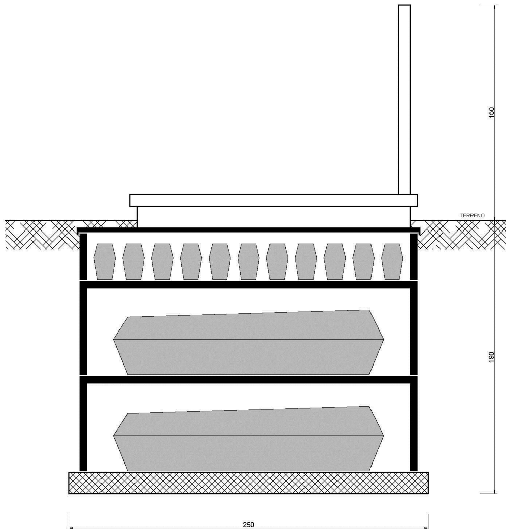
SEPOLCRO DI FAMIGLIA (TIPO A + TIPO B) VISTA LATERALE
